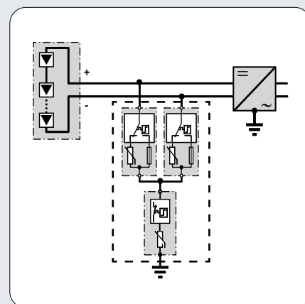
Schéma de principe DEHNGuard M YPV SCI... (FM)
