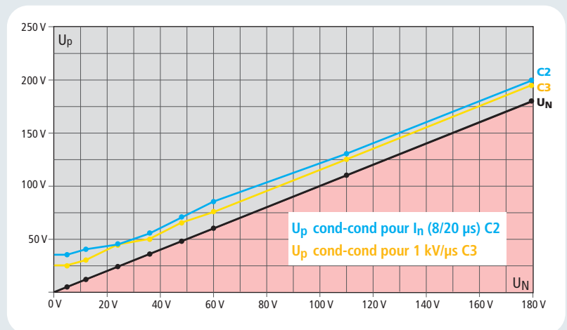
Diagramme du niveau de protection U_p
